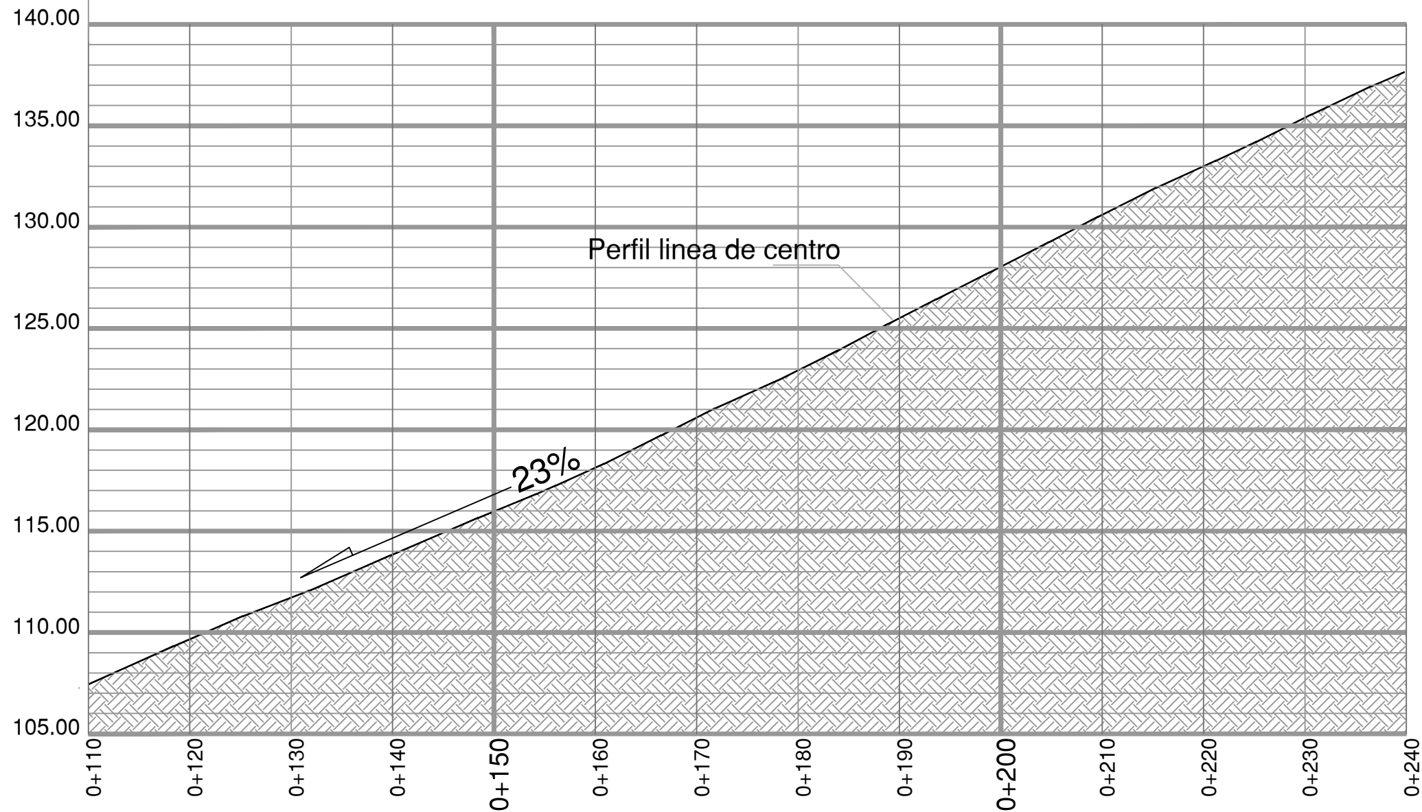
PERFIL TOPOGRAFICO ESCALA HORIZONTAL 1:500 VERTICAL 1:250
