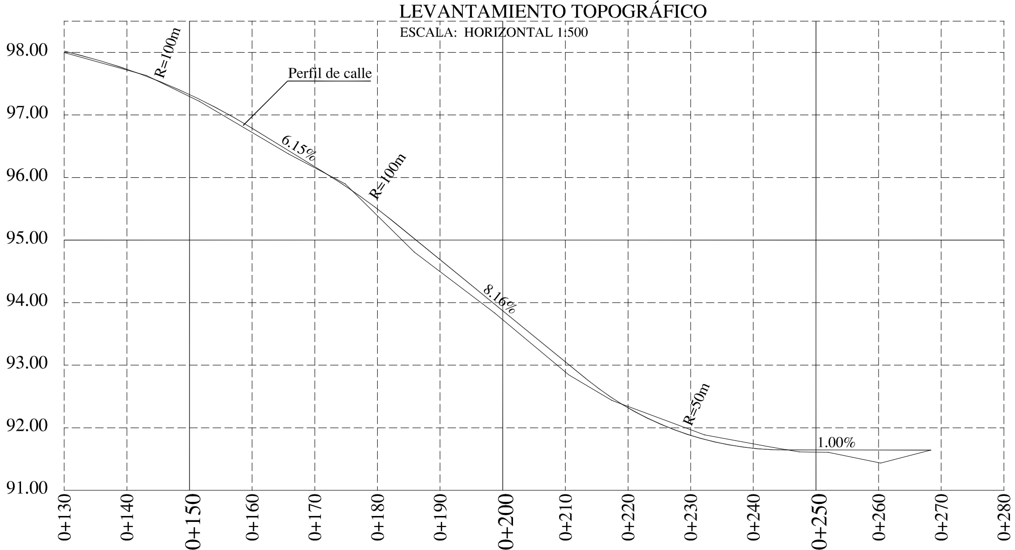
PERFIL TOPOGRAFICO LINEA DE CENTRO CALLE CAÑAS ESCALA: HORIZONTAL 1:500 VERTICAL 1:50
