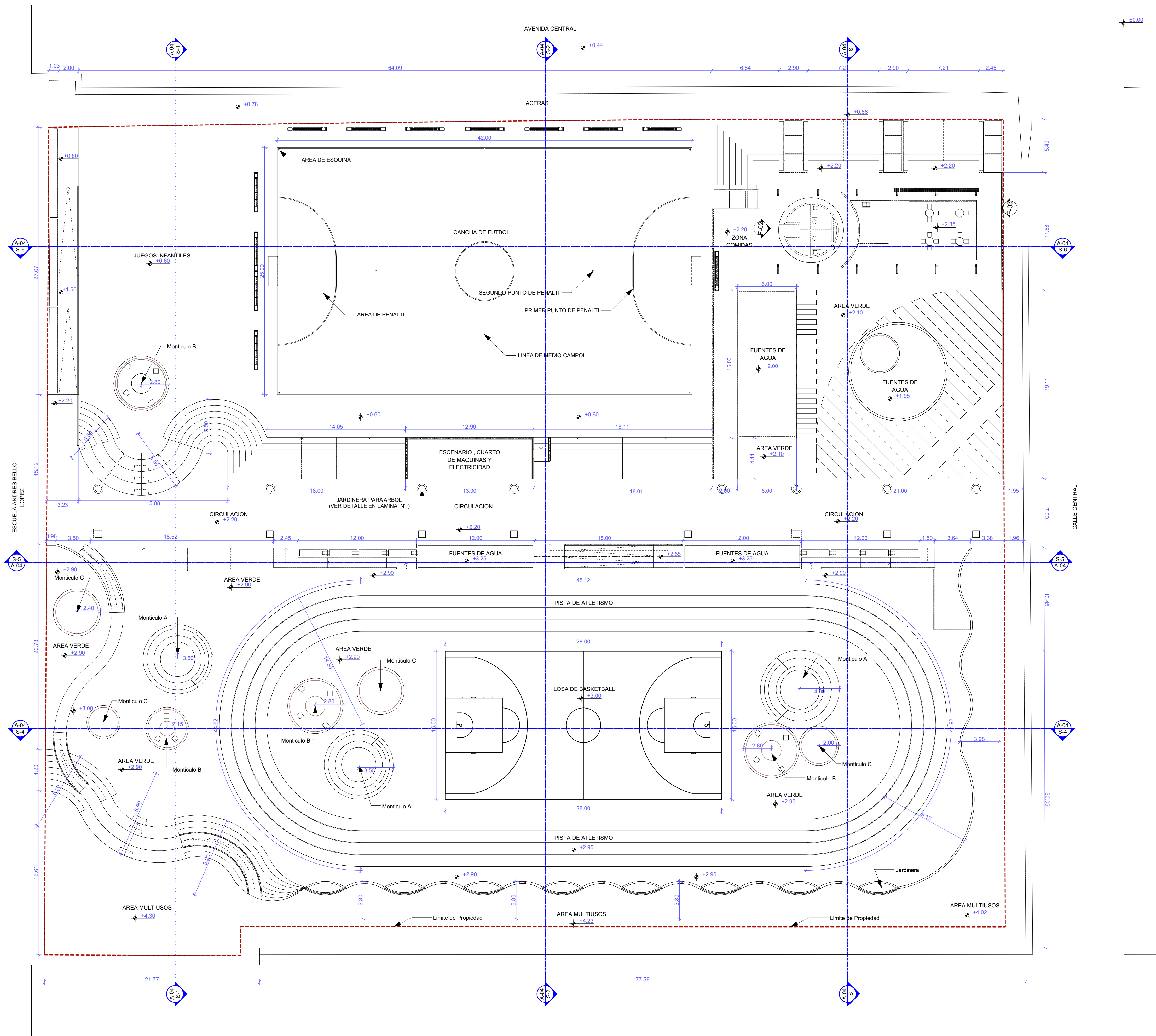
PLANTA CONJUNTO PROPUESTA ESCALA: 1/200
