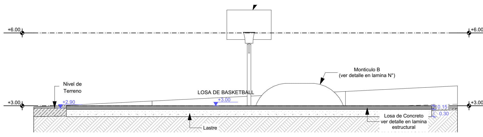
CORTE S-11 ESC=1:75
