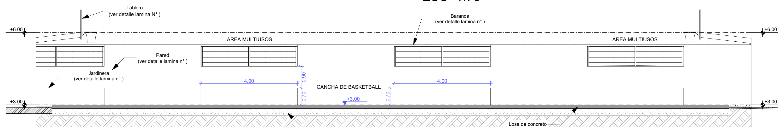
CORTE S-12 ESC=1:75
