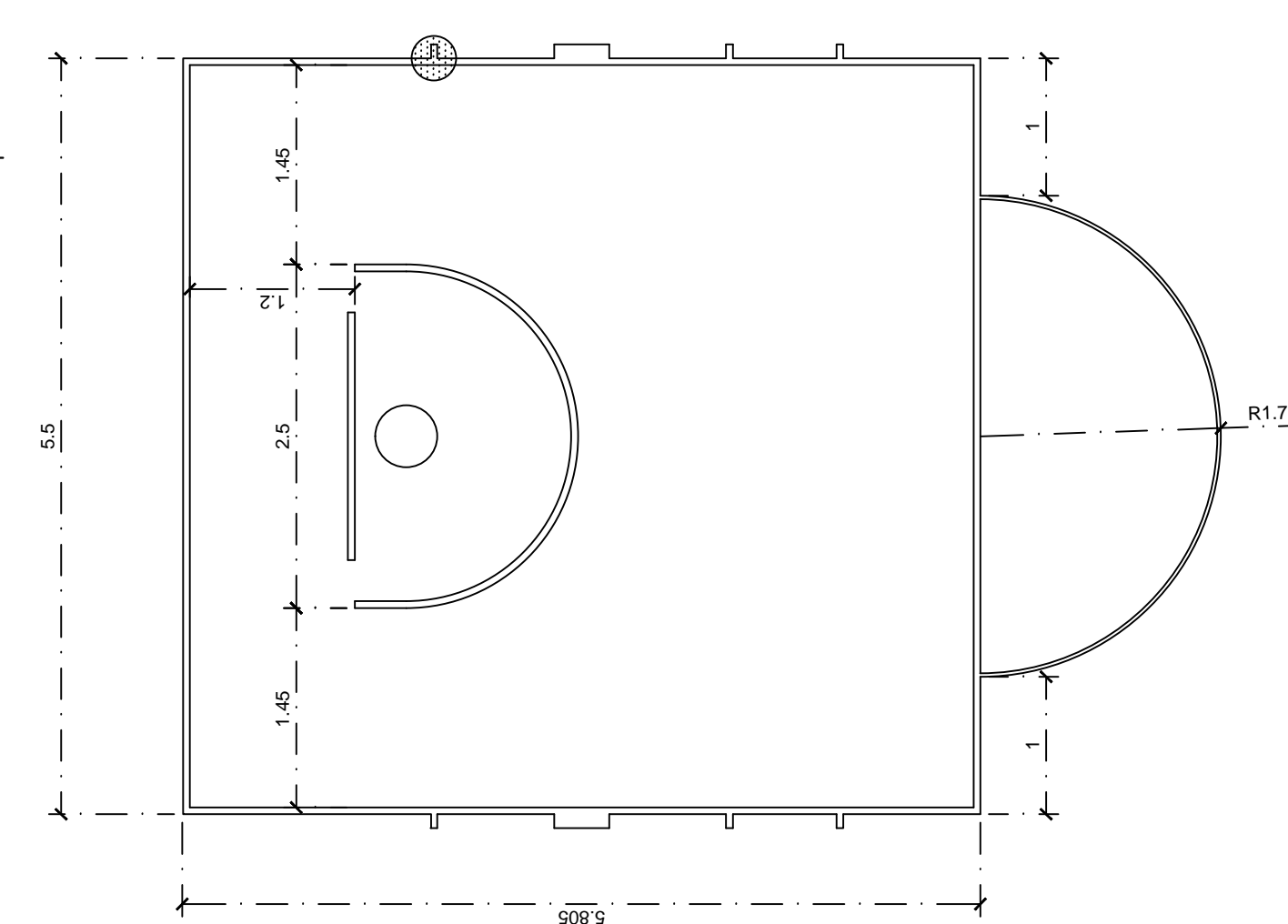
ZONA DE LANZAMIENTO ESC=1:50
