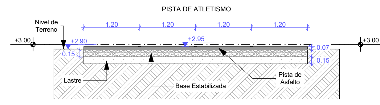
DETALLE 01 PISTA DE ATLETISMO ESC=1:50
