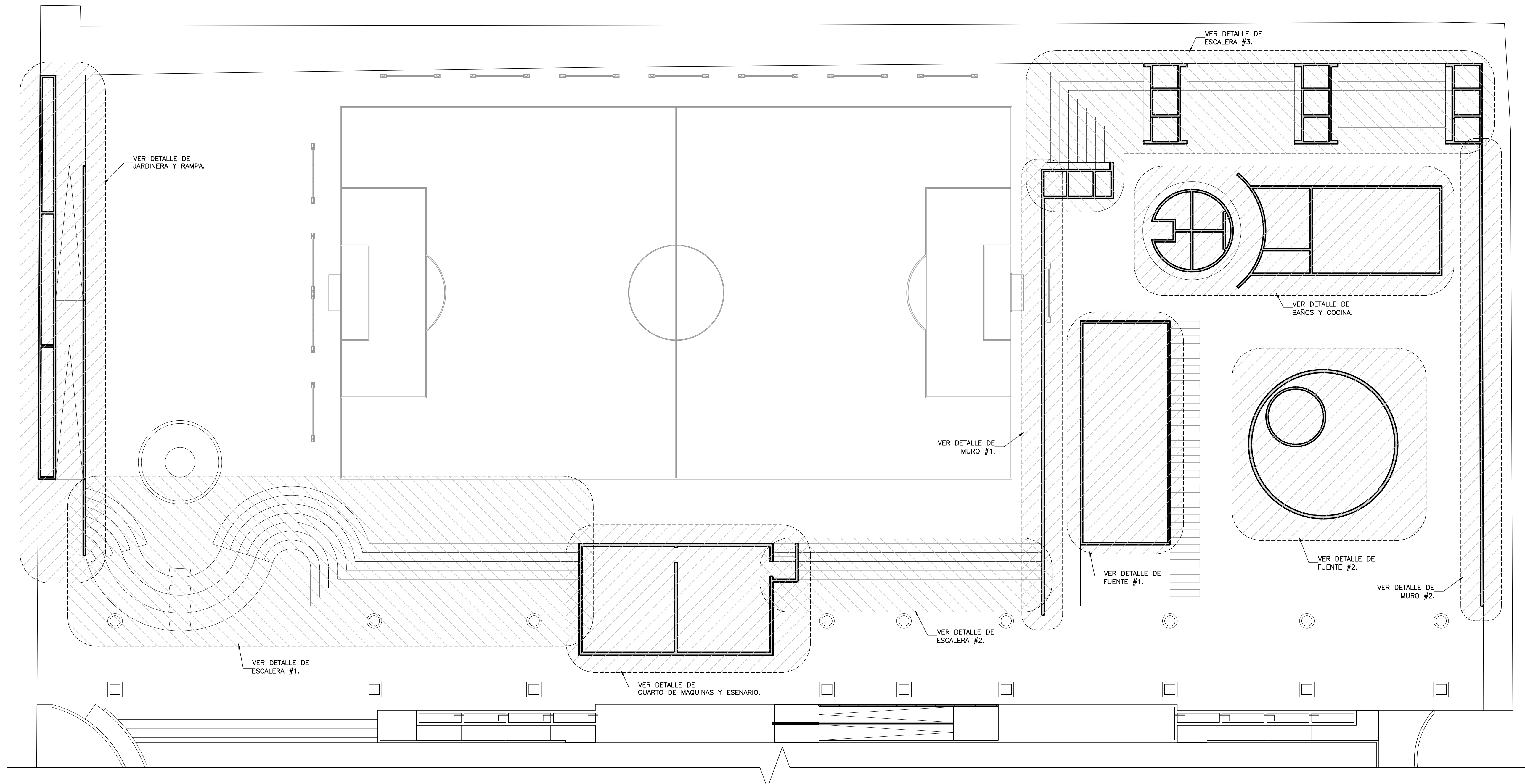
PLANTA ESTRUCTURAL DE UBICACION. ESCALA 1:150
