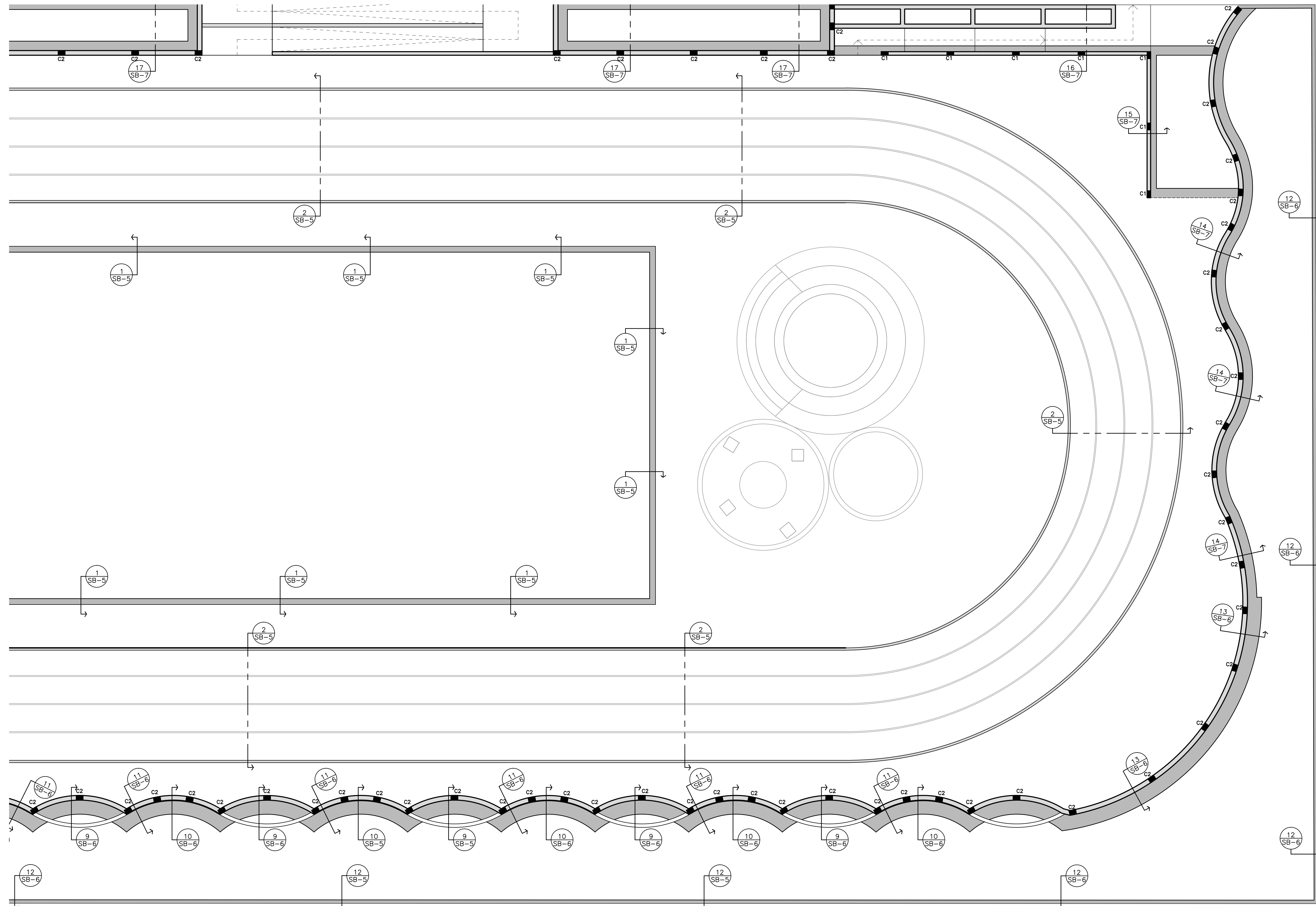
PLANTA ESTRUCTURAL DE FUNDACIONES Y COLUMNAS. ESCALA 1:75
